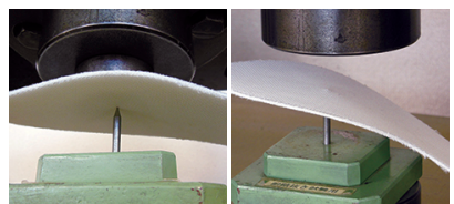
踏抜き性能試験
